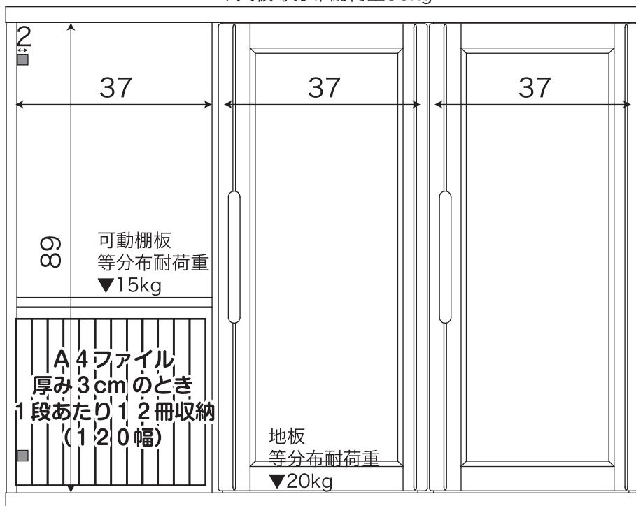
OF-120 開戸
