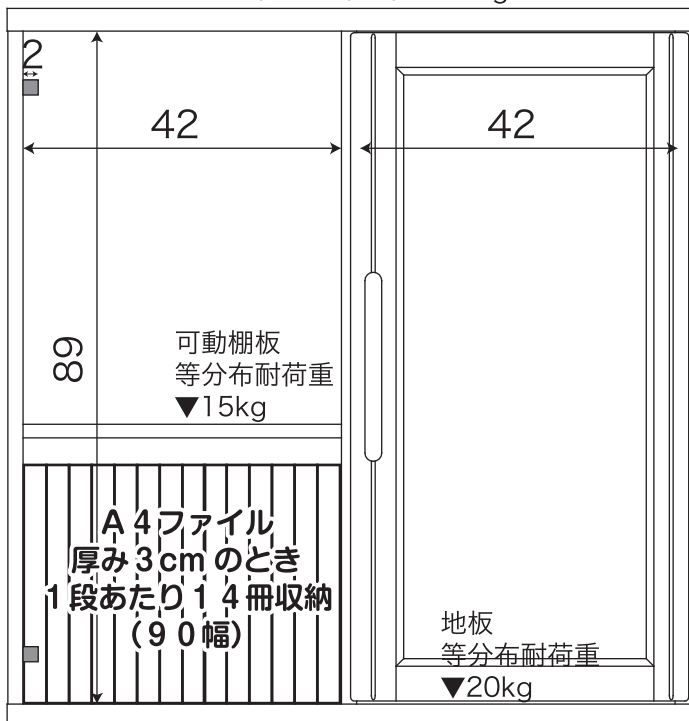
OF-90 開戸
